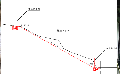
標準断面図
